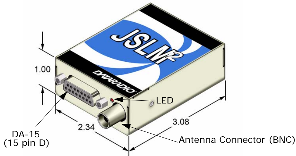
Figure 2-1 JSLM2 Module
